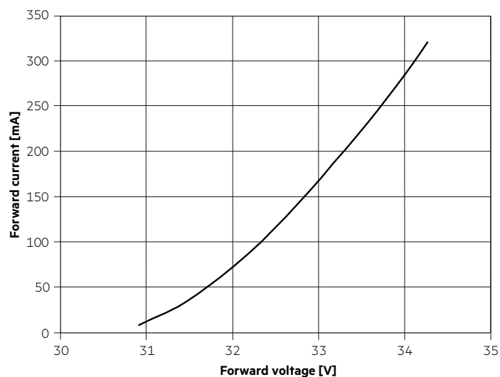
LLE 24x560mm 1300lm 9xx LV ADV5
