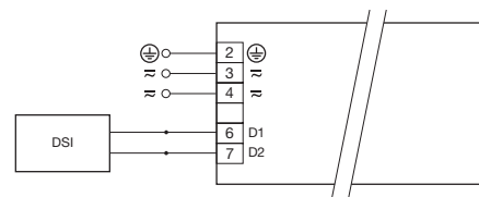
DSI PCA T5 BASIC Ip xrtec II
