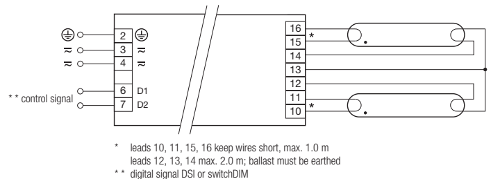
PCA T5 BASIC Ip xitec II 2x14–80 W
