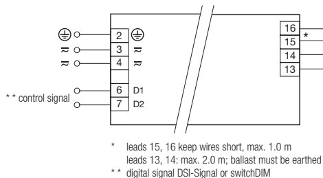
PCA T5 BASIC Ip xitec II 1x14–80 W
